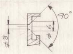
Snitt A-A
