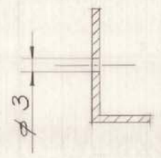
Snitt A-A
