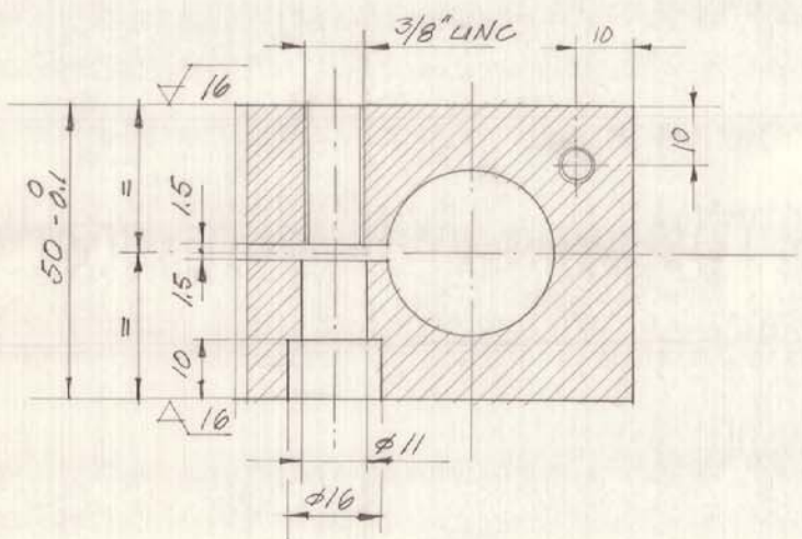
SNITT A-A
