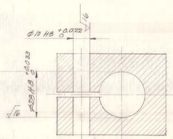
SNITT B-B
