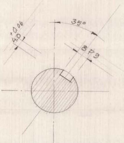
SNITT A-A SKALA 1:1
